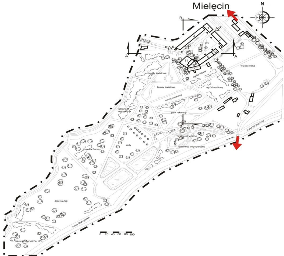
Rys. 3. Koncepcja zagospodarowania założenia pałacowo-folwarcznego w Zastrużu: 1, 2 – centrum SPA, 3 – zadaszony parking, 4 – śmietnik, 5 – hotel, 6, 7, 8, 9 – baza gastronomiczna, 10 – kaplica pałacowa, 11 – ruiny pałacu, 12 – budynek mieszkalny
