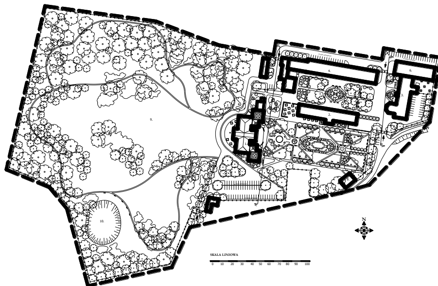
Rys. 1. Koncepcja zagospodarowania założenia pałacowo-folwarcznego w Mańczycach: 1 – centrum konferencyjne, 2 – centrum gastronomiczne, 3 – hotel, 4 – centrum sportowe, 5 – administracja, 6 – garaże, 7 – portiernia, 8 – budynek gospodarczy
