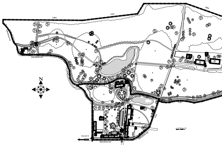
Rys. 2. Koncepcja zagospodarowania założenia pałacowo-folwarcznego w Świniarach: 1, 4, 5, 7, 8, 9, 11, 14, 19 – budynek mieszkalny, 2 – budynek inwentarski, 3, 12 – budynek gospodarczy, 6 – garaż, 10 – minizoo, 15, 16, 20 – wiata, 17 – stajnia, 13 – klub jeździecki
