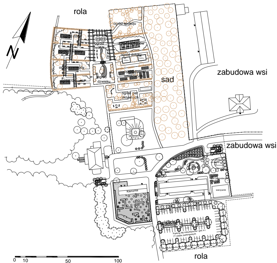
Rys. 4. Koncepcja zagospodarowania założenia pałacowo-folwarcznego w Królikowicach: 1 – pensjonat seniora, 2 – karczma, 3 – budynek mieszkalny Fig. 4. The concept of development of the mansion-grange complexes in Królikowice: 1 – a retirement home, 2 – an inn, 3 – a dwelling house
